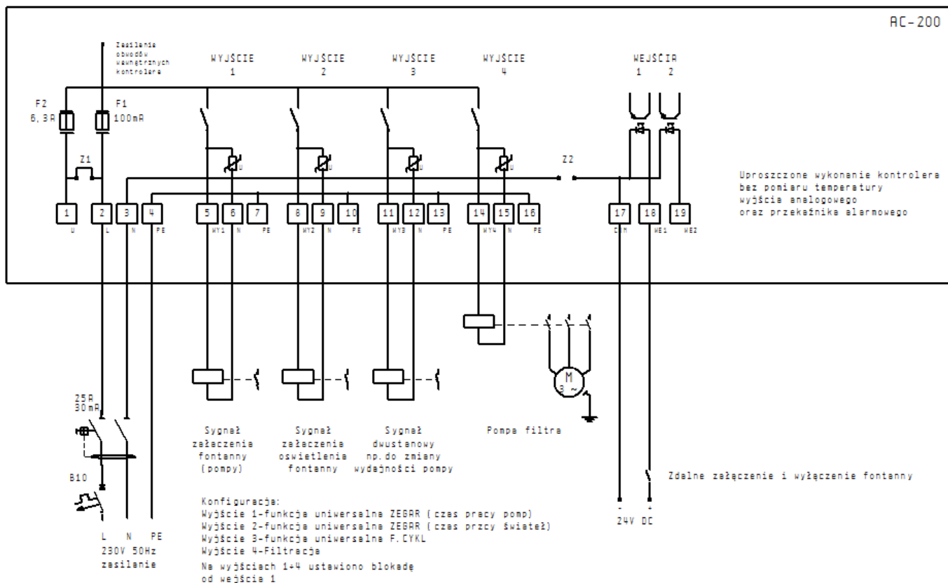
Rys. 4 Fontanna Funkcje: sterowanie pracą urządzeń fontanny, filtracja
