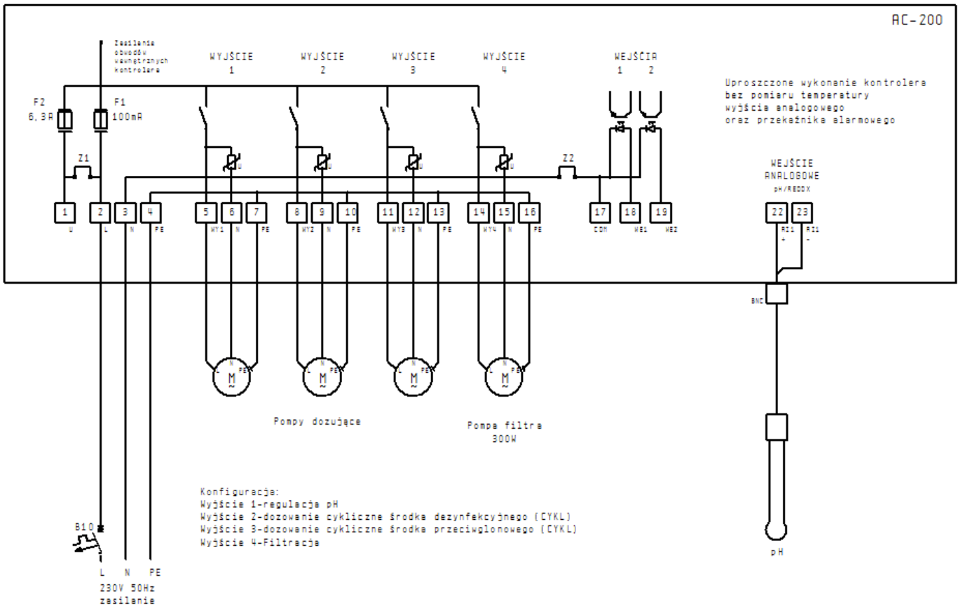
Rys. 2 Basen/fontanna Funkcje: dozowanie chemii, filtracja
