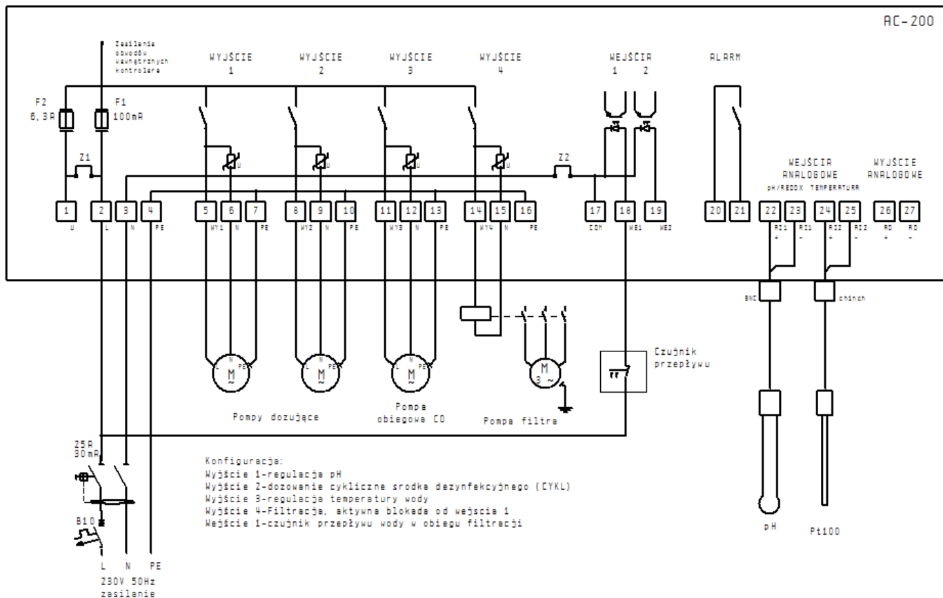
Rys. 3 Basen Funkcje: dozowanie chemii, ogrzewanie wody, filtracja
