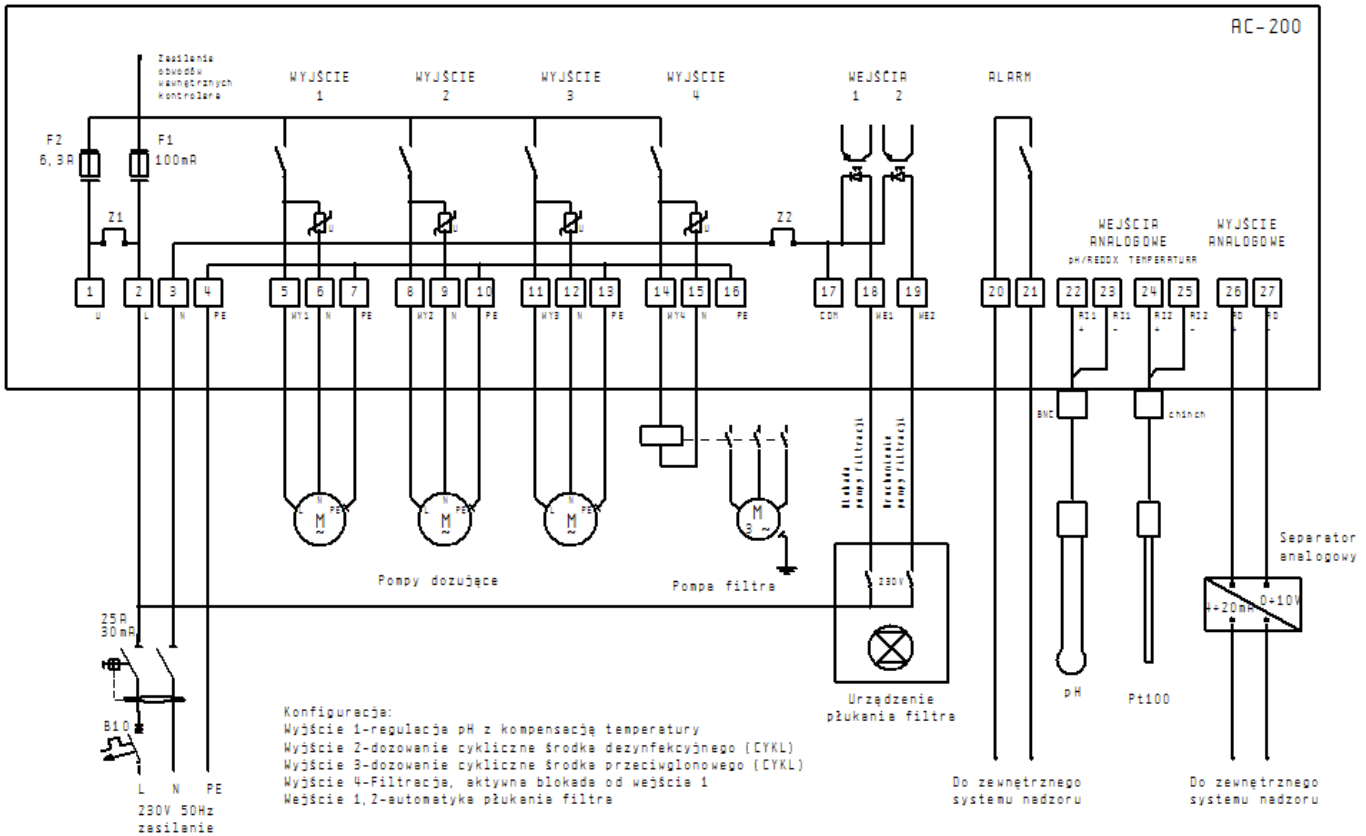
Rys. 1 Basen/fontanna Funkcje: dozowanie chemii, filtracja
